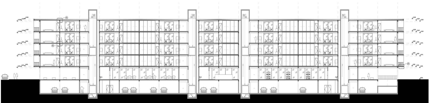
Corte A
