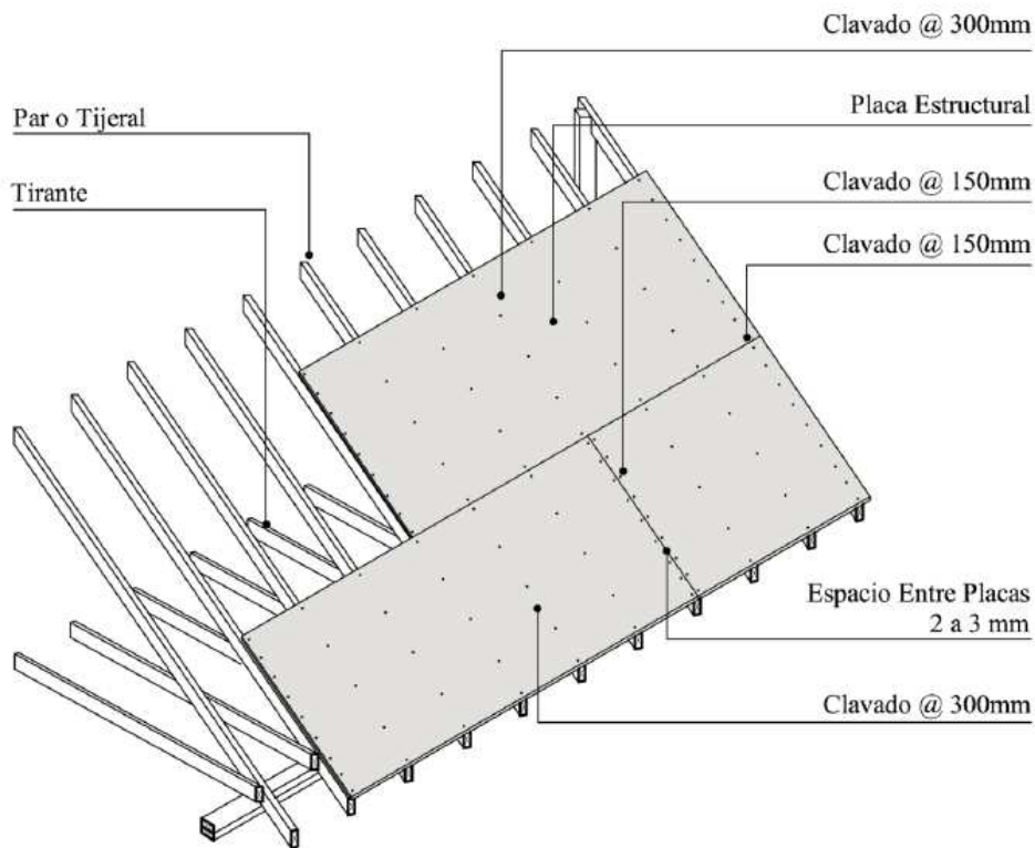
Figura 54. Colocación del diafragma de techumbre. Fuente: (González R, Vázquez V, & Hernández C, 2011)
