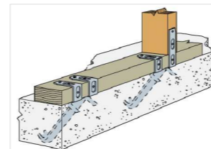
Conector MASZ StrongTie
