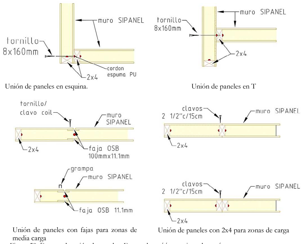
Figura 59: Formas de unión de paneles. Fuente: http://www.sipanel.com/
