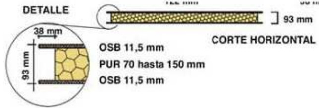
Figura 57. Detalles de conformación de aleros. Fuente: (González R, Vázquez V, & Hernández C, 2011)
