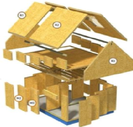
Figura 21: Despiece constructivo Fuente: http://www.sipanel.com
