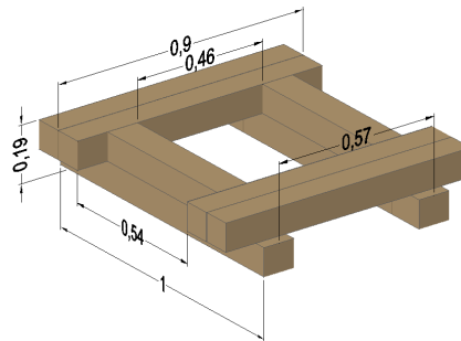
Figura 12. Pallet tipo II. Fuente elaboración propia
