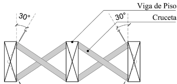
Figura 42. Instalación de arriostramiento cruzado. Fuente: (González R, Vázquez V, & Hernández C, 2011)
