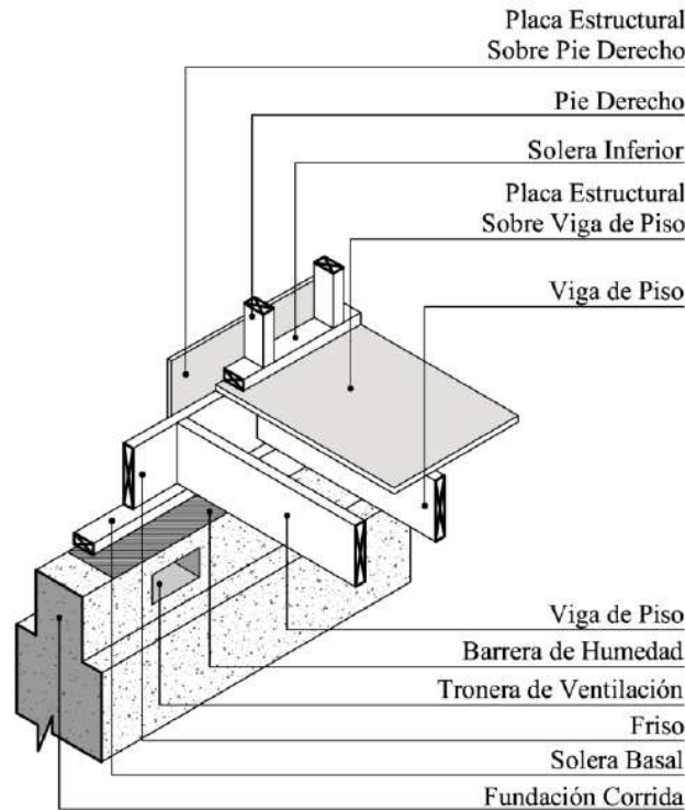
Figura 47: Encuentro de sobrecimiento corrido y envigado de piso Fuente: (González R, Vázquez V, & Hernández C, 2011)
