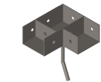
Base de esquina, anclaje de columna y soleras con pernos y tuercas autofrenante de 3/4"
