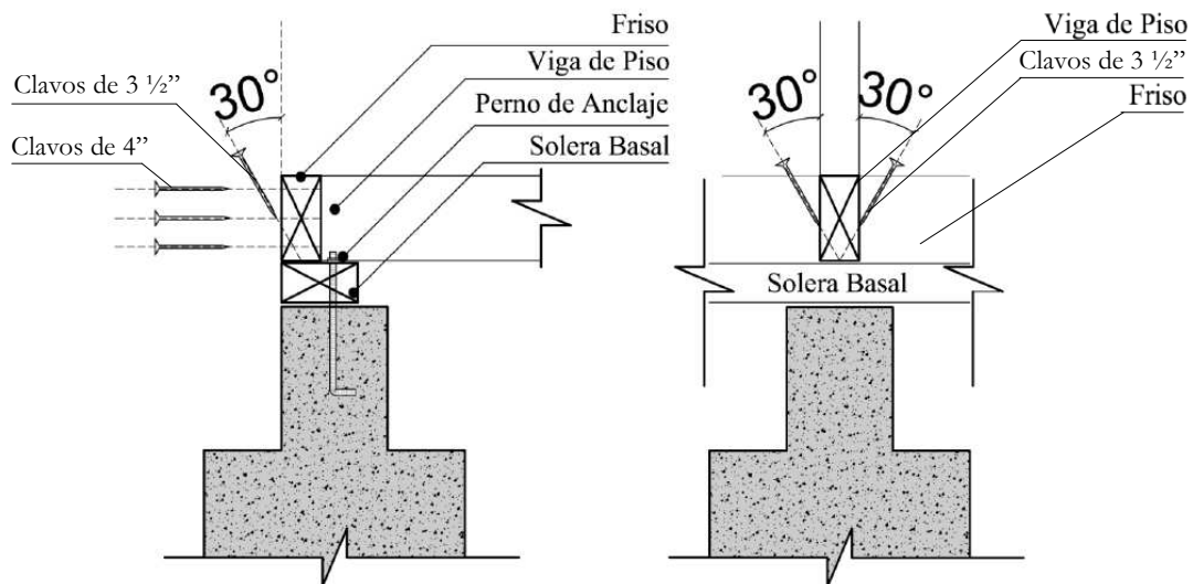
Figura 40. Fijación de las vigas de piso a la fundación corrida. Fuente: (González R, Vázquez V, & Hernández C, 2011)
