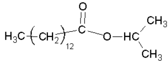
Figura 10. Estructura del Miristato de Isopropilo
